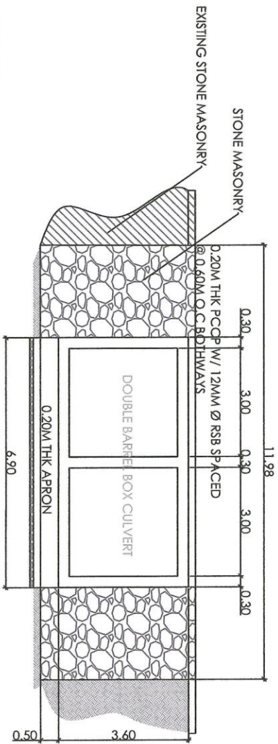
ELEVATION SCALE: NTS
