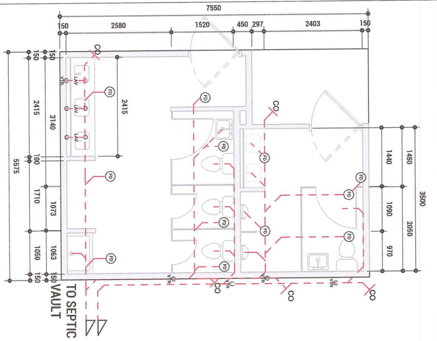
1 1 : 50 GF SEWERLINE LAYOUT
